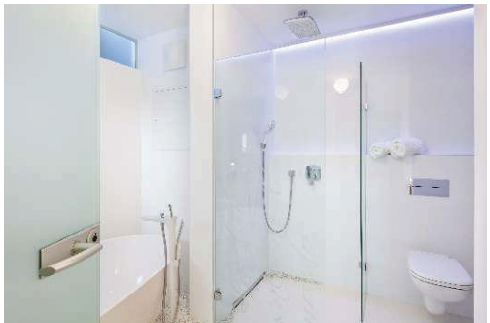
fixní sprchová zástěna 700/2000 mm + 800/2000 mm, sklo: Float čirý 8 mm s povrchovou úpravou proti usazování vodního kamene a zasychání vodních kapek, vzor: pískování - atyp, kování: Dorma BH 200
